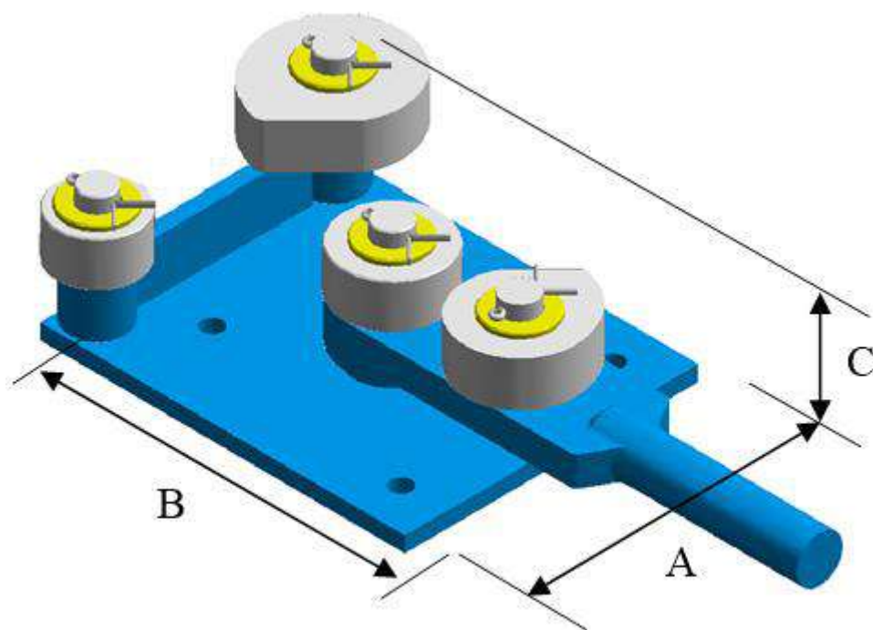
Размеры DR-25
