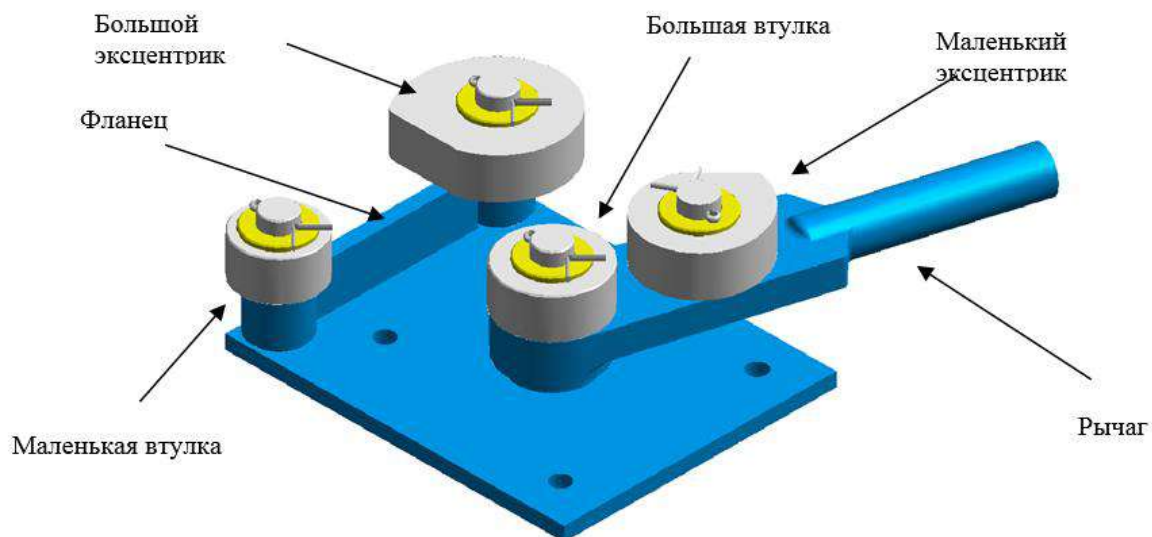
Детализовка гибочной машины DR-25
