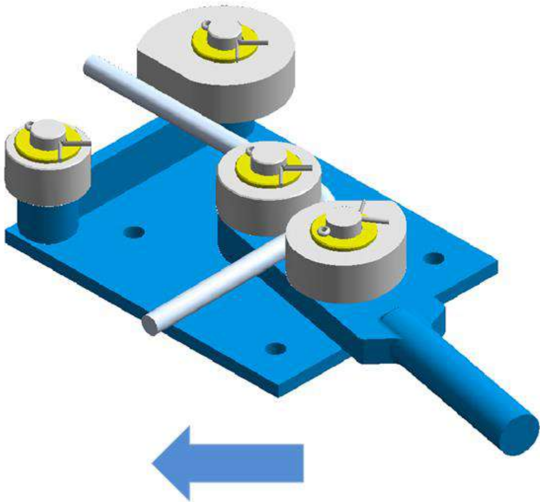
Прут, согнутый при помощи гибочных машин DR-25
