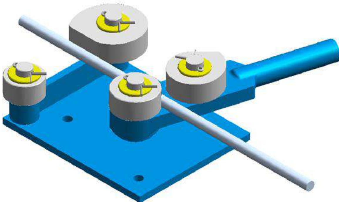
Расположение прута в гибочных машинах DR-25
